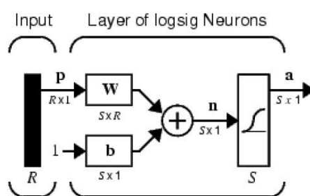
شکل (۲): معماری MLP
