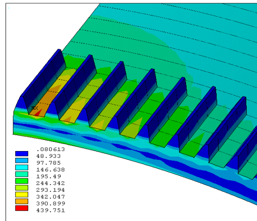
شکل (۱۳): طیف تغییرات تنش فون مایسز در ریشه‌ی دندانه به ازای L = 80 \text{ mm} و R = 663
