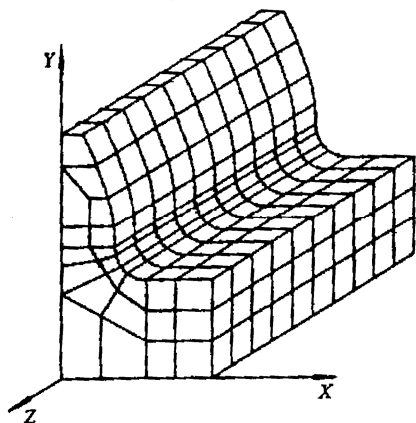
شکل ۶-ب: نمای المان بندی شده‌ی نیمی از یک دندانه‌ی متصل به پوسته‌ی انعطاف پذیر
