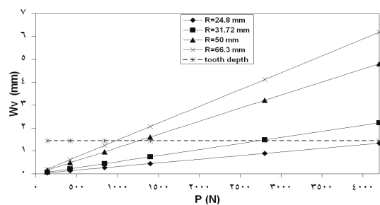
شکل (۱۰): جابجایی قائم ایجاد شده در دندانهای پوسته‌ی انعطاف پذیر به
