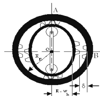
ه. موقعیت دندانه‌ها پس از بارگذاری
