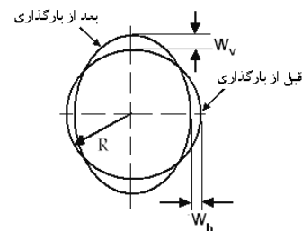
د. موقعیت چرخ‌دنده‌ی انعطاف پذیر قبل و بعد از بارگذاری
