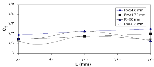
شکل (۸): منحنی تغییرات C_f بر حسب L
