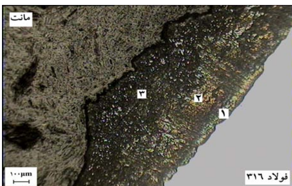
شکل (۵): ریزساختار پوشش فولاد زنگ نزن ۳۱۶ درون روی مذاب ۱ غوطه ور شده به مدت ۱۲۰ ساعت در دمای ۴۵۸°C (با استفاده از میکروسکوپ نوری)، نقطه ۱: فصل مشترک، نقطه ۲: دلتا، نقطه ۳: زتا
