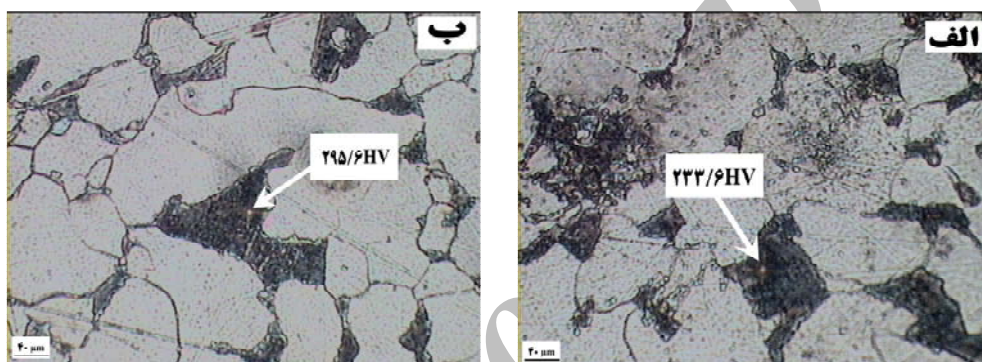
شکل (۷): سختی اندازه گیری شده برای فولاد ۱۰۱۵ (میکروسکوپ نوری) درون روی ۱ در دمای 458^{\circ}\text{C} درمرز پوشش - فولاد(سمت فولاد) الف) غوطه ور شده به مدت ۲۴ ساعت ب) غوطه ور شده به مدت ۱۲۰ ساعت
