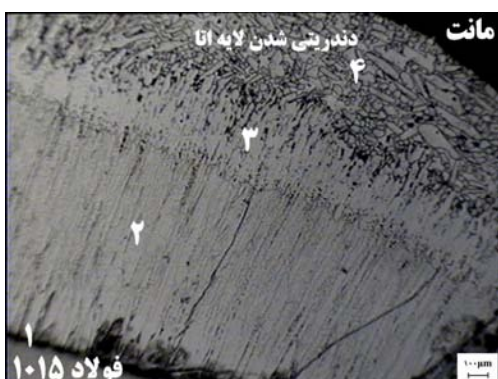
شکل (۲): ریزساختار پوشش ایجاد شده بر روی فولاد ۱۰۱۵ غوطه ور شده درون روی ۱ برای مدت زمان غوطه وری ۱۲۰ ساعت در دمای ۴۵۸°C (میکروسکوپ نوری). نقطه ۱: فصل مشترک، نقطه ۲: دلتا، نقطه ۳: زتا، نقطه ۴: اتا
