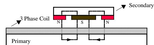
شکل ۷- ساختار یک بر با ثانویه کوتاه و آهنربای سطحی
