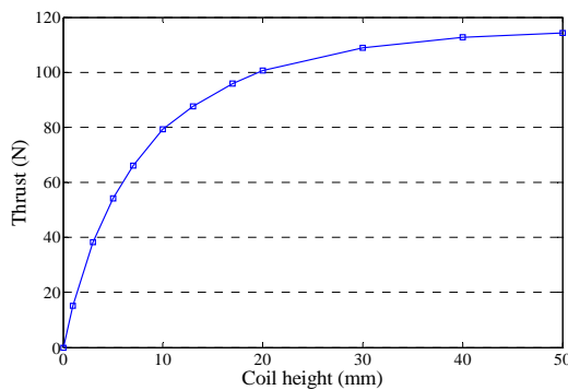
شکل ۳۰- تغییرات نیرو برحسب ارتفاع سیم‌پیچی
