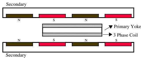
شکل ۱۴- ساختار دوپلر با دو ثابویه بلند با آهنربای درونی و یک اولیه کوتاه یوغ‌دار
