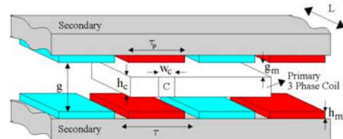
شکل ۲۵- ساختار یک موتور سنکرون آهنربای دائم خطی دو پیر با
