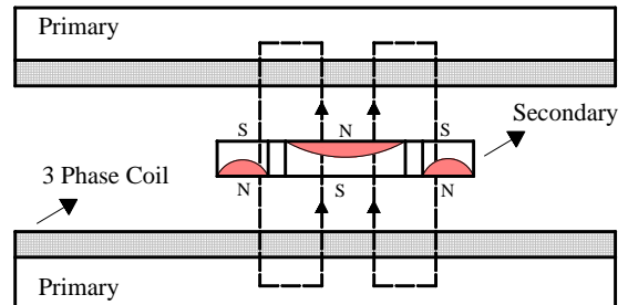
شکل ۲۳- ساختار دوپور با یک ثانویه کوتاه با آهنربای افقی و دو اولیه بلند
