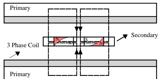
شکل ۲۴- ساختار دوپور با یک ثانویه کوتاه با آهنربای عمودی و دو اولیه بلند
