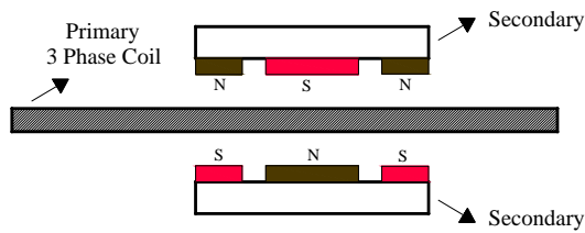
شکل ۱۹- ساختار دوبر با دو ثانویه کوتاه با آهنربای سطحی و یک اولیه بلند با هسته هوایی
