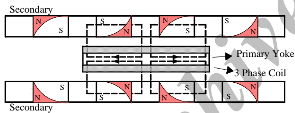
شکل ۱۵- ساختار دوپلر با دو ثابویه بلند با آهنربای درونی عمودی و اولیه کوتاه یوغ‌دار
