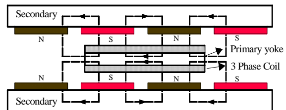
شکل ۱۲- ساختار دوپلر با دو ثابویه بلند با آهنربای سطحی و یک اولیه کوتاه یوغ‌دار
