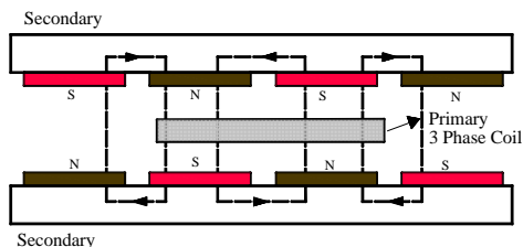
شکل ۱۱- ساختار دوبر با دونانویه بلند و یک اولیه کوتاه با هسته
