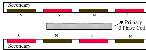
شکل ۱۳- ساختار دوپلر با دو ثابویه بلند و یک اولیه کوتاه با هسته هوایی و آهنربای درونی
