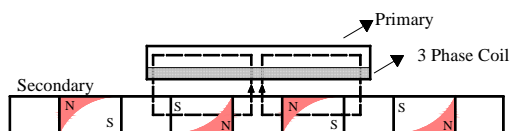
شکل ۶- ساختار یک بر با اولیه کوتاه و آهنربای درونی عمودی
