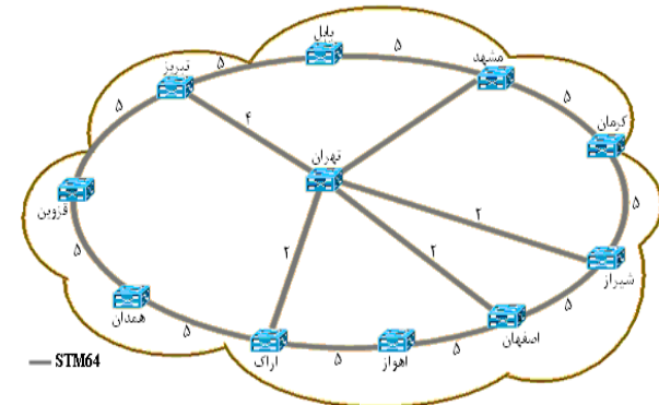
شکل ۲- همبندی پیشنهادی شبکه داده در سطح لایه هسته
