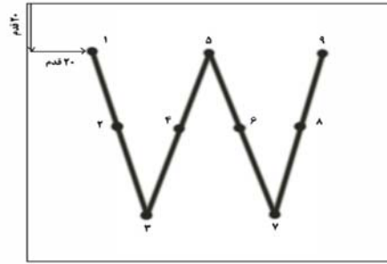
شکل ۲- روش نمونه‌گیری در مزرعه (توماس، ۱۹۹۱)
