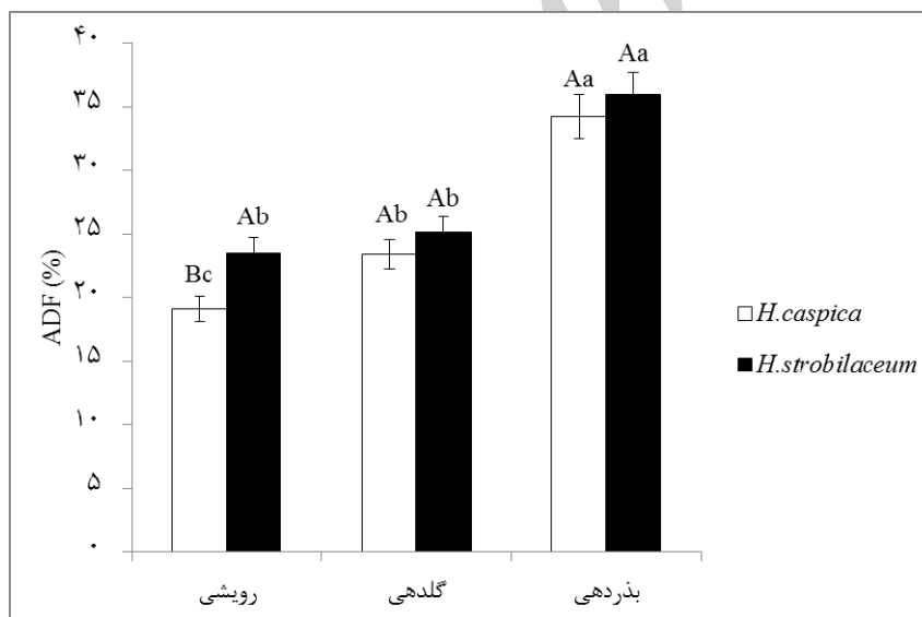
شکل ۲- میانگین ( \pm انحراف معیار) درصد ADF گونه‌های مورد مطالعه در مراحل مختلف فنولوژیک حروف کوچک نشان دهنده معنی داری یا عدم معنی داری در بین مراحل مختلف فنولوژیکی است و حروف بزرگ معنی داری یا عدم معنی داری بین گونه‌ها را نشان می‌دهد
