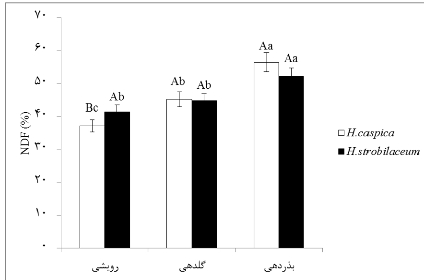
شکل ۳: میانگین (± انحراف معیار) درصد NDF گونه‌های مورد مطالعه در مراحل مختلف فنولوژیک
