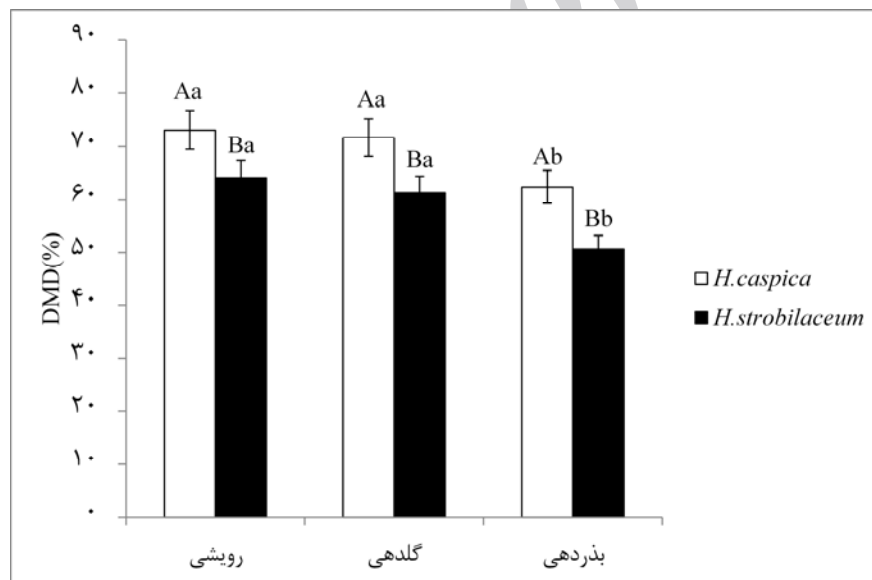
شکل ۴- میانگین (± انحراف معیار) درصد DMD گونه‌های مورد مطالعه در مراحل مختلف فنولوژیک
