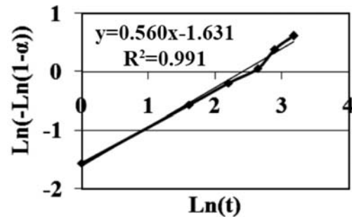
شکل ۴. مطالعه سینتیکی بازیابی مس از غبار با استفاده از باکتری های مزوفیل در دمای ۳۵ °C.
