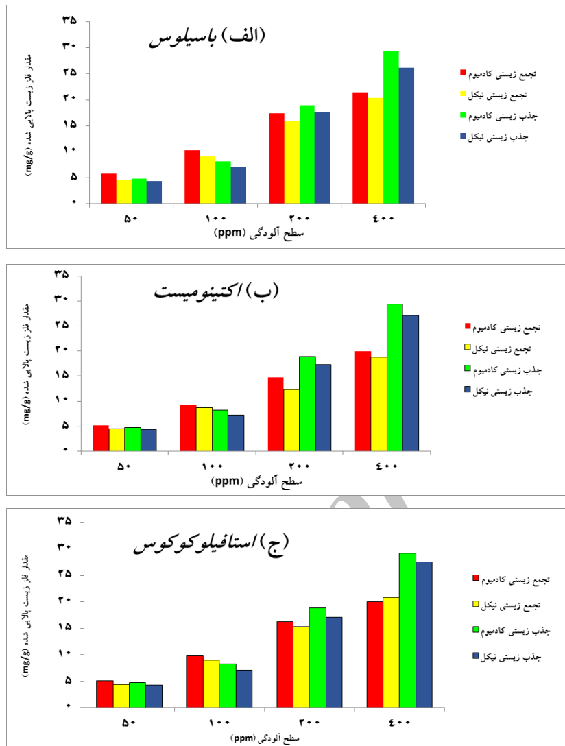
نمودار ۱: مقدار تجمع زیستی و جذب زیستی کادمیوم و نیکل توسط (الف) باسیلوس، (ب) اکتینومیسیت و (ج) استافیلوکوکوس.
