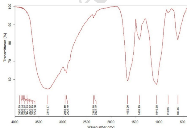
شکل ۷: طیف FTIR نانوذرات مس تولید شده توسط رومانند کشت باسیلوس لیکنی فورمیس سویه Cu25.
