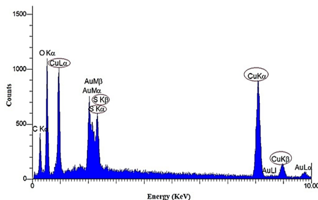
شکل ۶: طیف EDX نانوذرات مس تولید شده توسط رومانند کشت باکتری باسیلوس لیکنی فورمیس سویه Cu25.
