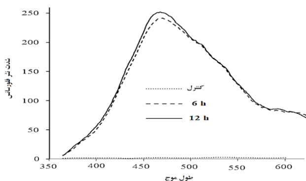
شکل ۲: طیف‌های نشی فلورسانس محلول‌های سولفات مس (غلظت یون مس ۵ میلی‌مولار، pH برابر ۷)، بدون رومانند (قسمت A) و به دنبال اضافه کردن رومانند کشت سویه Cu25 (قسمت B)، پس از ۶ و ۱۲ ساعت واکنش زیست تبدیلی در ۲۵ درجه سلسیوس روی شیکر مدور (۱۵۰ دور در دقیقه).
