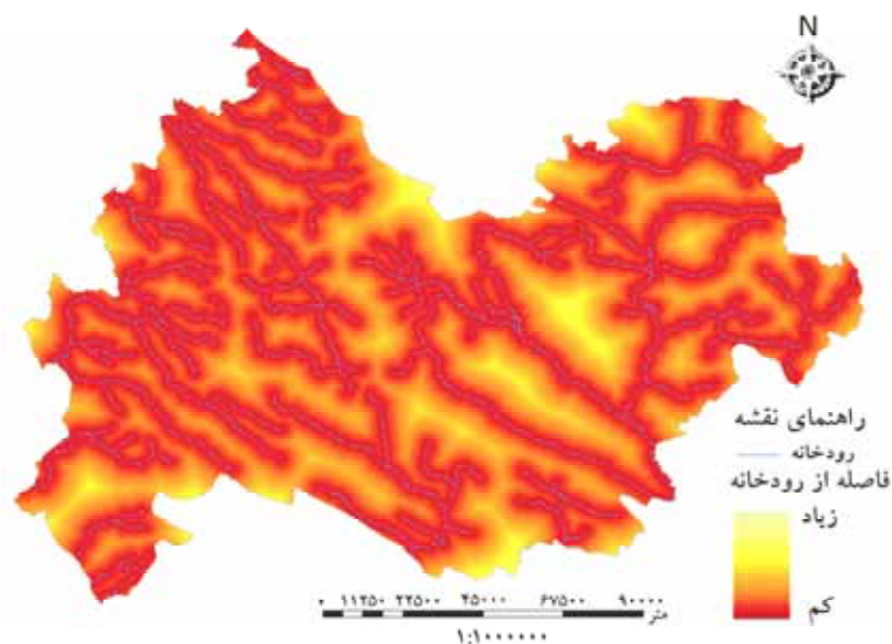
شکل ۴. رودخانه‌های استان کرمانشاه و فواصل متعدد از آن‌ها
