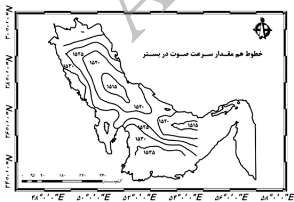
شکل ۱۲. خطوط هم مقدار سرعت صوت (m/s)، بستر خلیج فارس در فصل گرم
