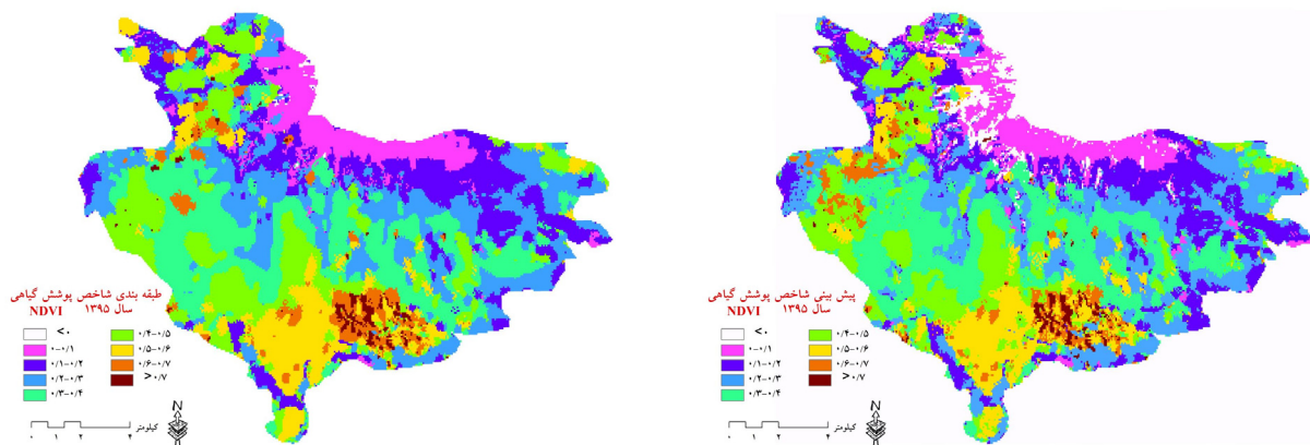
شکل ۷. مقایسه شاخص NDVI سال ۱۳۹۵ (سمت چپ) و پیش بینی توسط مدل مارکوف سال ۱۳۹۵ (سمت راست)
