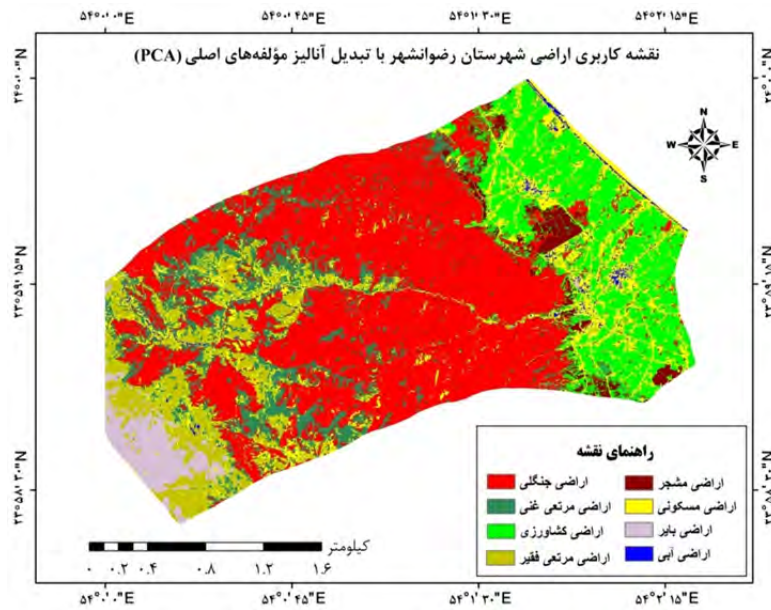
شکل ۴. نتایج حاصل از طبقه بندی خروجی تبدیلی آنالیز مؤلفه های اصلی با ۸ کلاس کاربری
