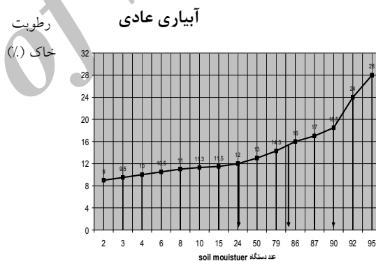
شکل ۱ - منحنی کالیبراسیون آبیاری
