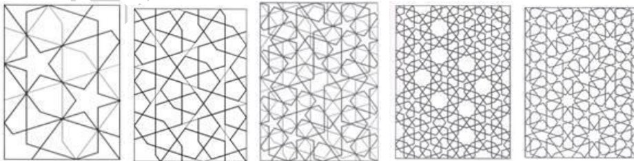
شکل ۳- اگر در یک زمینه گره «کند دو پنج» رسم کنیم و سپس بر اساس خصوصیت تکرار و
