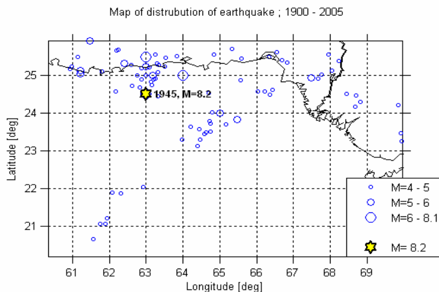
شکل ۹- نقشه توزیع جغرافیایی زمینلرزه های رخ داده در محدوده ۲
