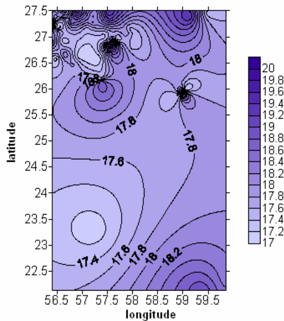
شکل ۷- منحنی های انرژی آزاد شده در محدوده اول از سال ۱۹۶۴ تا سال ۲۰۰۵
