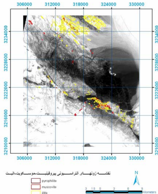
شکل ۴- نقشه زونهای دگرسانی پیروفلایت- موسکویت- ایلت
