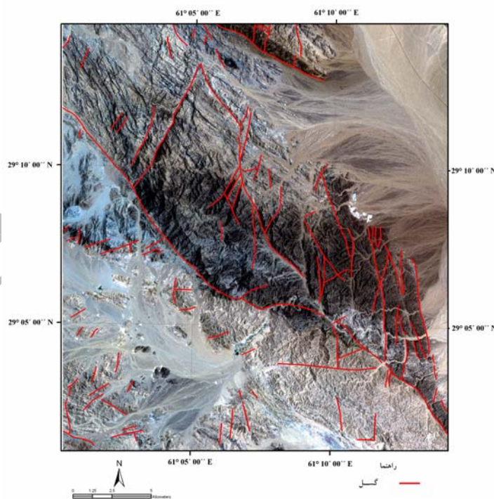
شکل ۳- گسل‌های مشخص شده بر روی عکس ماهواره‌ای منطقه
