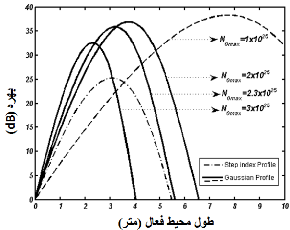
شکل ۸. تغییرات بهره در طول تقویت‌کننده. منحنی‌های پر معرف نمایه گوسی با بیشینه 2 \times 10^{25} ، 2.3 \times 10^{25} و 3 \times 10^{25} یون بر متر مکعب را نمایش می‌دهند. دو منحنی رسم شده در شکل ۱ با توان پمپاژ ۱۰ میلی‌وات برای مقایسه با منحنی‌های خط چین رسم شده‌اند.
