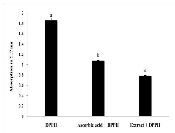
شکل ۱. کاهش جذب رادیکال آزاد DPPH در حضور اسید آسکوربیک و عصاره S. aethiopsis
