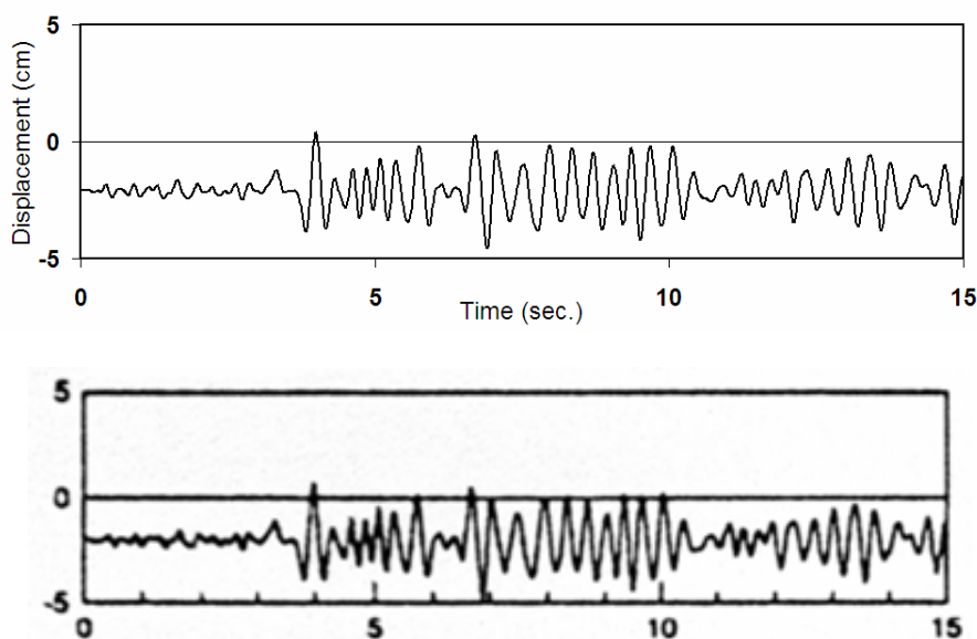
نمودار ۸ پاسخ تاریخچه زمانی سد ماروپوینت به زلزله Taft با در نظر گرفتن تمامی اثرات اندرکنشی (نمودار بالایی) و مقایسه روش پیشنهادی با یکی از پژوهش‌های پیشین و شناخته شده [۱۳] (نمودار پایینی)
