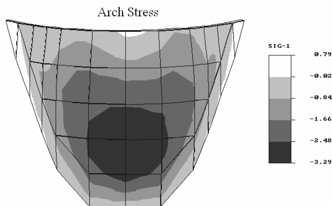
نمودار ۹ دیگرام پوش تنش‌های اصلی (با واحد مگاپاسگال) در وجه بالادست سد ماروپوینت به خاطر اعمال زلزله Taft و با در نظر گرفتن تمامی اثرات اندرکنشی
