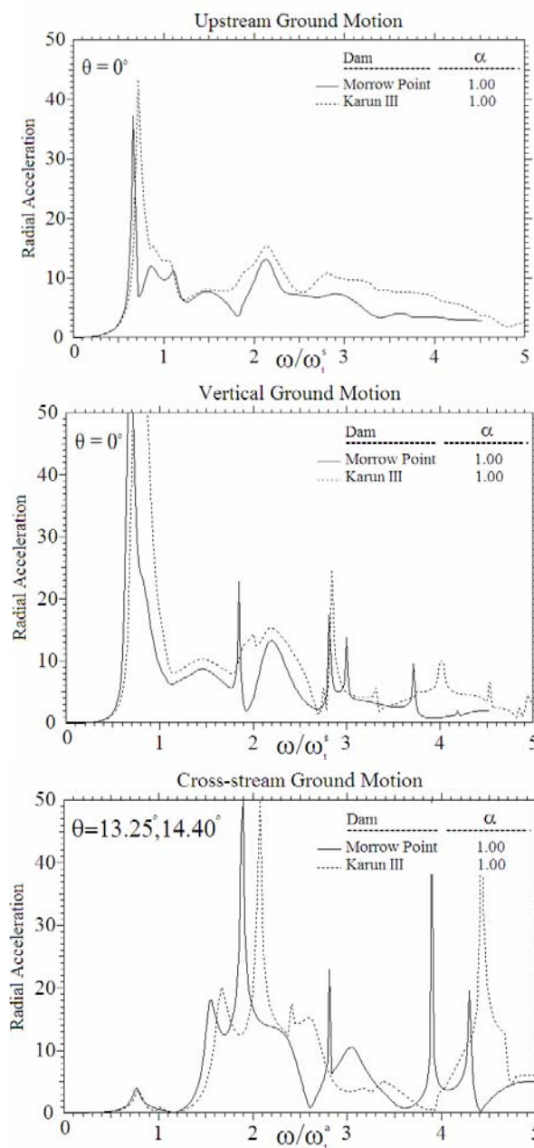
نمودارهای ۶ مقایسه توابع پاسخ فرکانسی دو سد، با مخزن پُر و \alpha=1 بر حسب فرکانس نرمال شده نسبت به فرکانس مودهای اول هر یک از دو سد قوسی در حالت مخزن خالی
