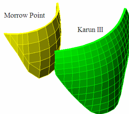
شکل ۱ مقایسه ظاهری دو سد قوسی ماروپوینت و کارون ۳
