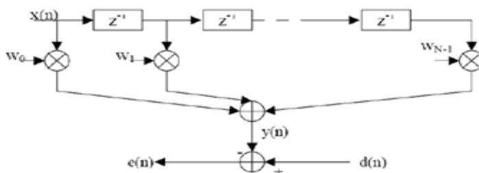
شکل (۲): فرآیند الگوریتم LMS و فیلترینگ عرضی
