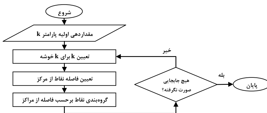
نمودگر ۶- مراحل کلی تکنیک K-means
