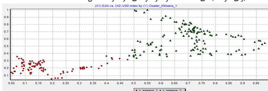
نمودگر ۹- نمایش تخصیص داده ها به دو خوشه
