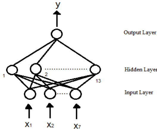
شکل ۱- ساختار ۱-۱۳-۷ شبکه عصبی
