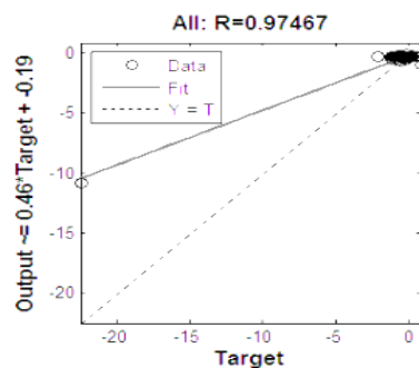
نمودار ۳- ضریب همبستگی کل شبکه عصبی
