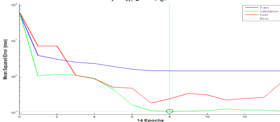
نمودار ۴- روند تغییرات خطای mse شبکه
