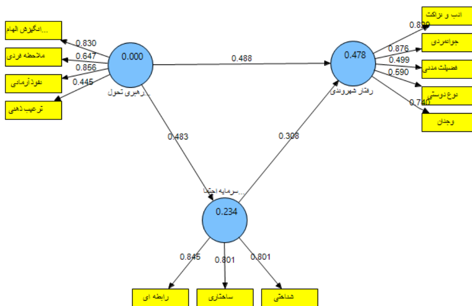
شکل ۲: مدل اندازه‌گیری
