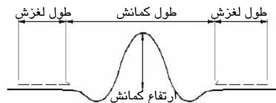
شکل ۲ - نواحی مختلف در یک کمانش مود ۳
