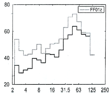
شکل ۳: مقایسه نتایج محاسبات (منحنی سیاه رنگ) با آزمایش (منحنی خاکستری رنگ) که محور قائم کمیت مجذور میانگین مربعات (rms) مربوط به سرعت زره با واحد دسی بل (با مقدار مرجع 10e-8 ) و محور افقی فرکانس می باشد
