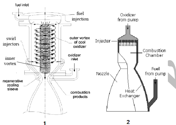
شکل (۱): نمای شماتیک محفظه احتراق گردابه ای (۱)
