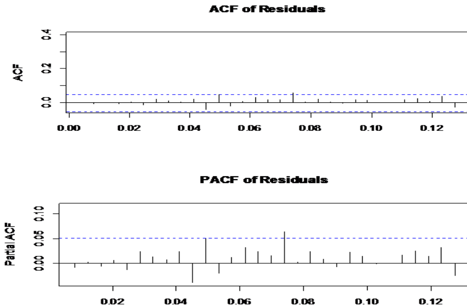
نمودار (۲): توابع همبستگی و همبستگی جزئی جملات پسماند مدل SETAR از نرخ بازده
