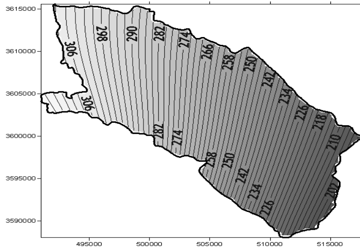
شکل ۵- نقشه همباران حوضه آبریز موسی آباد تیران
