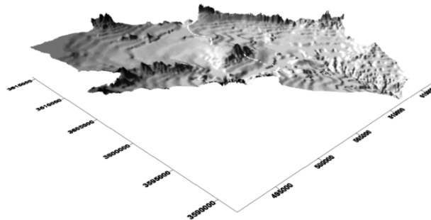
شکل ۱- نقشه سه بعدی حوضه آبریز موسی آباد تیران
