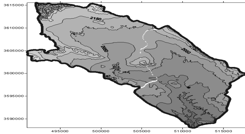
شکل ۲- نقشه توپوگرافی حوضه آبریز موسی آباد تیران
