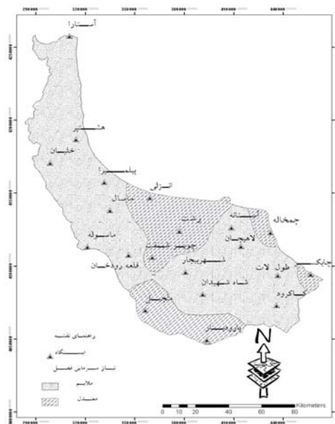
شکل ۶. میانگین مجموع درجه/ روزهای مورد نیاز سرمایش (CDD) فصل تابستان در استان گیلان
