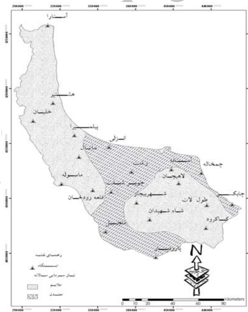
شکل ۳. میانگین مجموع درجه/ روزهای مورد نیاز سرمایش (CDD) سالانه در استان گیلان
