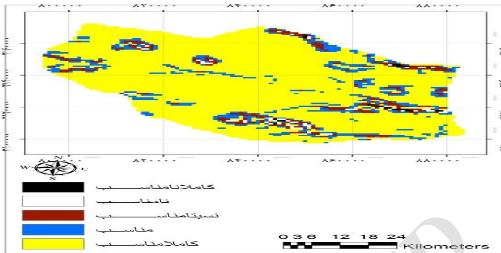
شکل ۴. لایه شیب
