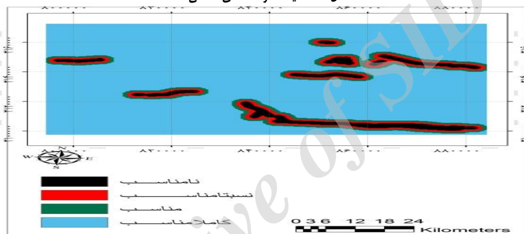
شکل ۱۱. لایه گسل
