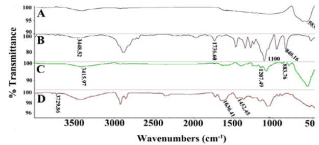
شکل ۳. طیف FT-IR (A) نانو ذرات Fe_3O_4 ، (B) COOH-PEG ، (C) نانو ذرات Fe_3O_4 / COOH-PEG ، (D) COOH-PEG لود شده با سیس پلاتین می باشد.
