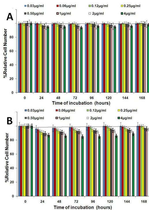
شکل ۱. مقایسه اثر سمیت، لوتشیم-۱۷۶ (A) و لوتشیم-۱۷۷ (B) در غلظت های مختلف در سلول های SKBR3
