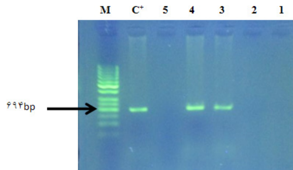
شکل ۲- کنترل مثبت همراه جواب PCR دو تا از نمونه‌های حاوی ژن czt (در چاهک ۳ و ۴، نمونه‌های سودوموناس آئروژینوزا، چاهک ۶، کنترل مثبت و چاهک ۷، مارکر)
