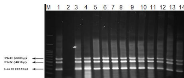
شکل ۱: نتایج واکنش PCR برای شناسایی ژن‌های ویروانس، راهک M-مارکر ۱۰۰ bp (فرمتاز)، راهک ۱- کنترل مثبت، ۲- کنترل منفی، راهک‌های ۳-۱۴
