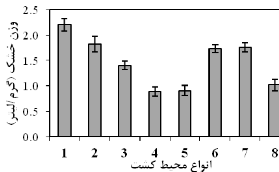
شکل ۲: مقایسه میزان رشد میسلیم قارچ شی تا که در محیط مایع (g/L): MMN -۱، PGC-۲، -۳ PGC+ویتامین B1، -۴ BM، -۵ BM +ویتامین B1، -۶ BM+CaCl 2 ، -۷ PDC، و -۸ PDC +ویتامین B1. تعداد تکرارها در این آزمایش ها بین ۳ تا ۵ تکرار برای هر نمونه بود. بر روی هیستوگرام بیانگر SD است.
