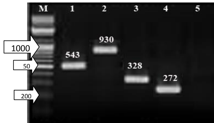
شکل ۳- ژل حاصل از الکتروفورز محصول PCR مربوط به ژن های cnf2 (قطعه ۵۴۳ جفت بازی)، PAI (قطعه ۹۳۰ جفت بازی)، papC (قطعه ۳۲۸ جفت بازی) و kpsMTHI (قطعه ۲۷۲ جفت بازی)، ستون M= مارکر ۱۰۰ جفت بازی DNA، ستون ۵= کنترل منفی
