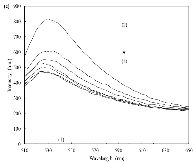
شکل ۳- تغییرهایی در نشر DNA با افزایش غلظت (a) نانوذرات دی اکسید تیتانیوم بدون پوشش ویژه، (b) نانوذرات دی اکسید تیتانیوم حاوی پایدارکننده \text{HNO}_3 و (c) نانوذرات دی اکسید تیتانیوم حل شده در ماتریکس پراکنده اتیلن گلیکول در دمای 37^\circ\text{C} درجه سانتی-گراد. (۱) نشر DNA، (۲) نشر DNA+DNA Green Viewer و (۳-۸) خاموشی نشر با افزایش غلظت نانوذرات دی اکسید تیتانیوم (۳-۱۹ میکرومولار)
