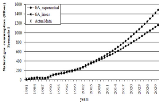
شکل ۱. مقایسه مدل های GA exponential و GA linear بر اساس سناریوی ۱.
