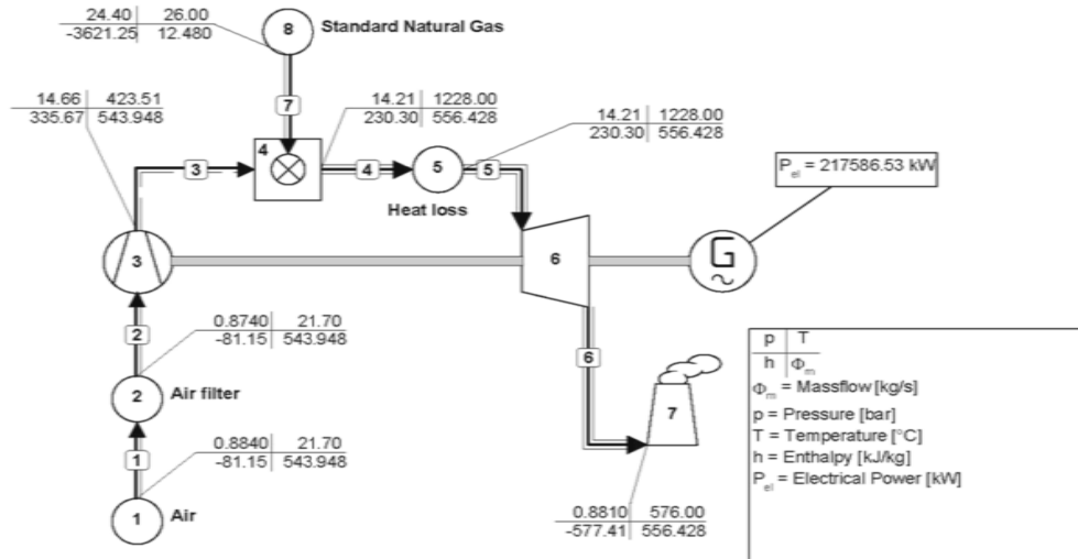
شکل ۱- سیکل شبیه سازی شده در بار ۱۰۰٪
