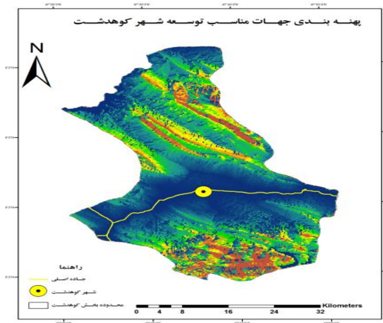
شکل ۵: نقشه نهایی حاصل از همپوشانی نقشه‌ها
