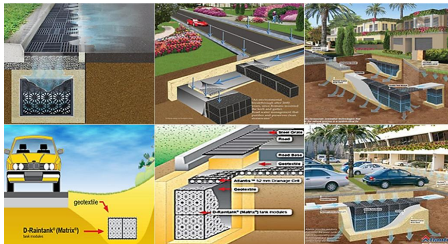
شکل ۱: موقعیت شبکه زهکش مسطح و مخازن CVF؛ مأخذ: بازسازی نگارندگان از شرکت ماناصنعت، ۱۳۹۴
