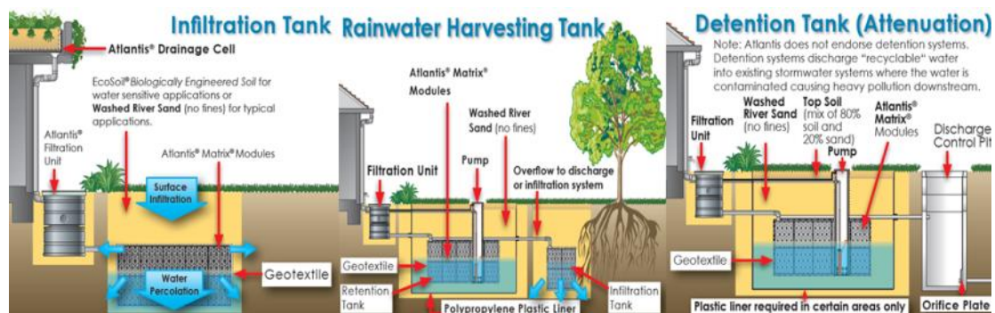
شکل ۲: موقعیت مخازن ذخیره‌سازی و استفاده مجدد از آب باران؛ مأخذ: شرکت آتلانتیس، ۲۰۱۴
