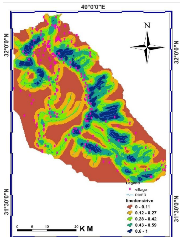
لایه فازی سازی شده تراکم زهکشی
