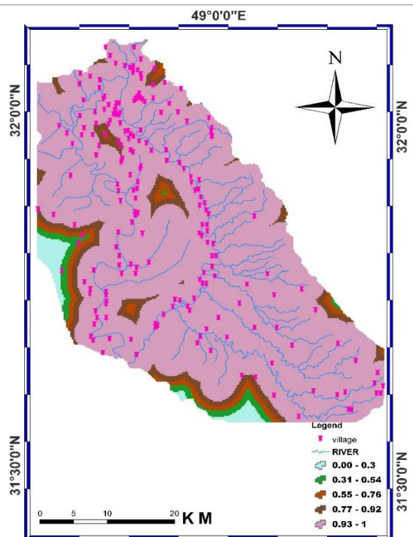
لایه فازی سازی شده فاصله از رودخانه
