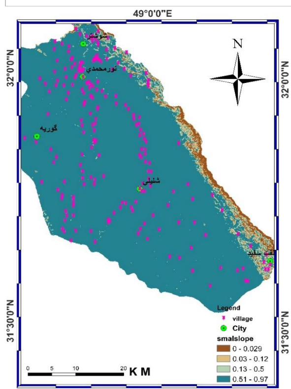
لایه فازی سازی شده شیب
