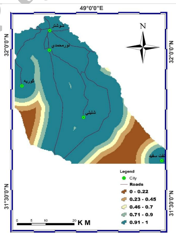
لایه فازی سازی شده فاصله از راه ارتباطی
