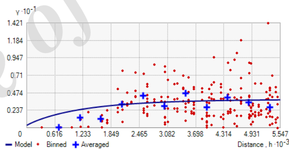
شکل ۸- مدل سمی واریوگرام پارامتر درصد رس
