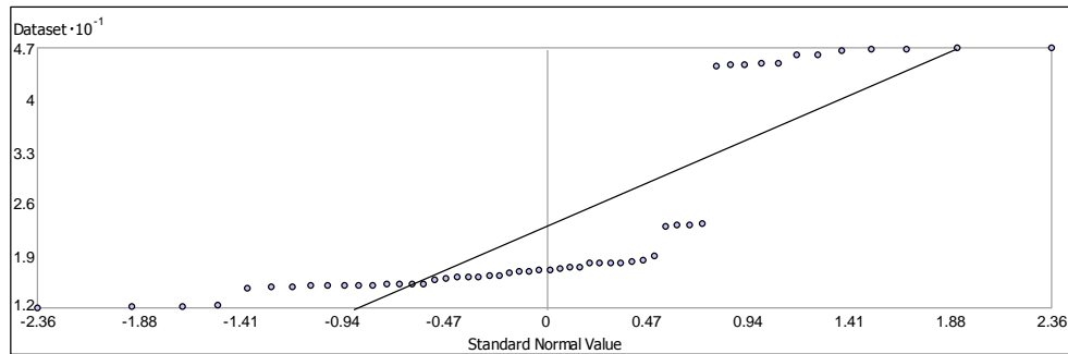
شکل ۴- گراف Q-Q Plot برای داده‌های درصد شن
