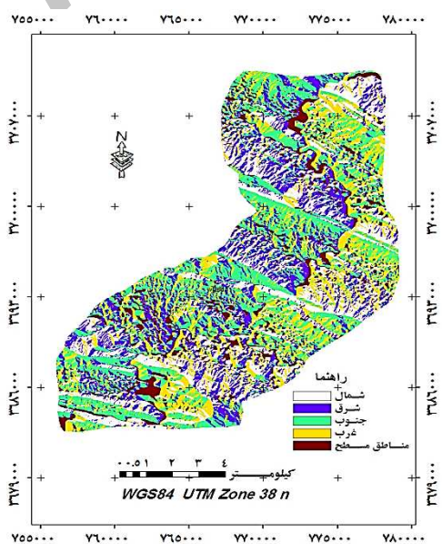
شکل ۵. نقشه طبقات جهت دامنه پراکنش ارغوان در منطقه پل دختر
