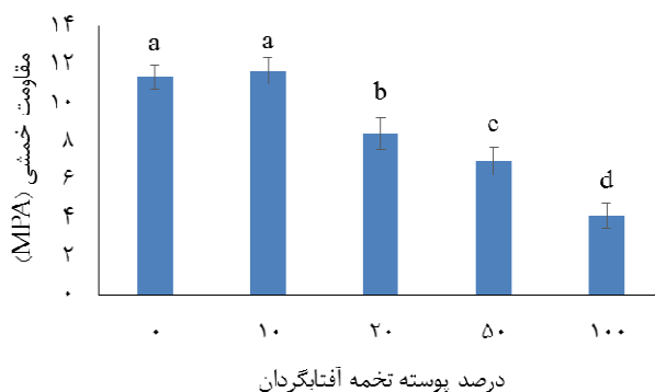
شکل ۱. تاثیر درصد پوسته تخمه آفتابگردان بر مقاومت خمشی (MOR) تخته‌خرده‌چوب ساخته شده از اختلاط پوسته تخمه آفتابگردان و خرده‌چوب صنوبر
