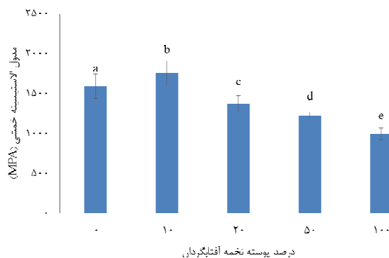
شکل ۲. تاثیر درصد پوسته تخمه آفتابگردان بر مدول الاستیسیته خمشی تخته‌خرده‌چوب ساخته شده از اختلاط پوسته تخمه آفتابگردان و خرده‌چوب صنوبر
