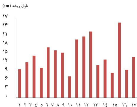
شکل ۳- نمودار مقایسه میانگین صفت طول ریشه نهال رملیک در اثر متقابل فاکتورهای مورد بررسی در آزمایش
