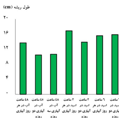
شکل ۴- نمودار مقایسه میانگین صفت طول ریشه نهال رملیک در اثر متقابل فاکتورهای مورد بررسی در آزمایش
