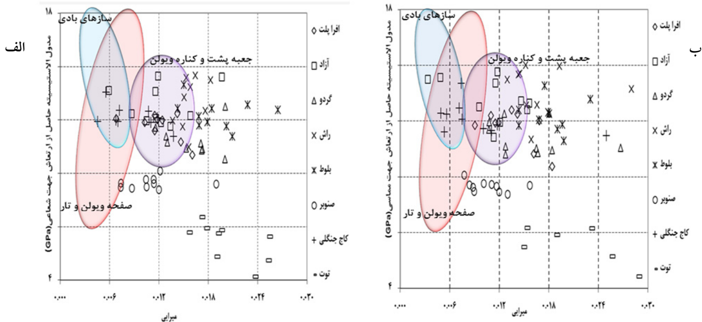
شکل ۴. معیار انتخاب چوب مناسب جهت هر بخش از ساز مطابق با مدول الاستیسیته و میرایی - جهت شعاعی (الف) جهت مماسی (ب)
