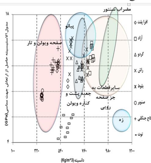
شکل ۳. معیار انتخاب چوب مناسب برای هر بخش از ساز مطابق با مدول الاستیسیته و دانسیته- جهت شعاعی (الف) جهت مماسی (ب)
